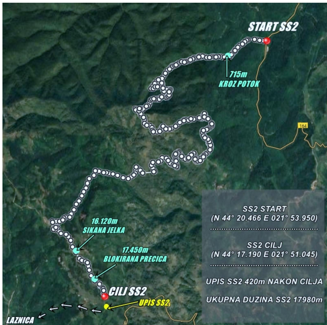
Skica Specijalnog ispita SI 2 – Zdravča 1
